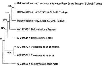
Şekil 20. Belone belone bireylerinin 12S rRNA gen bölgesi kullanılarak Komşu Birleştirme Metodu (Neighbor Joining) ile oluşturulmuş filogenetik ağaç.
