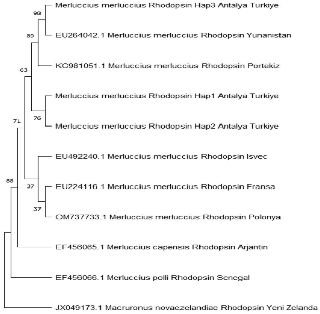
Merluccius merluccius bireylerinin Rhodopsin gen bölgesi kullanılarak Maksimum Benzerlik Metodu (Maximum Likelihood) ile oluşturulmuş genetik ağaç.
