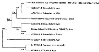
Şekil 17. Belone belone bireylerinin 16S rRNA gen bölgesi kullanılarak Maksimum Benzerlik Metodu (Maximum Likelihood) ile oluşturulmuş filogenetik ağaç
